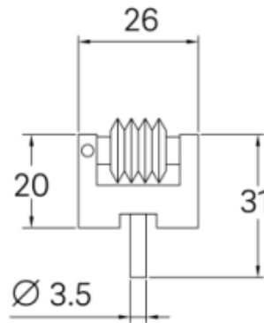
60° metrisch / 60° metric
